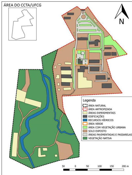
Figura 7 - Mapa de uso e ocupação atual do solo na Fazenda Experimental do CCTA/UFCCG.
